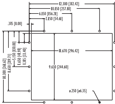
4612T Cutout
